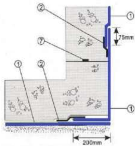
Oszlop részletterv
