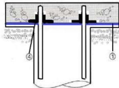
Oszlop részletterv
