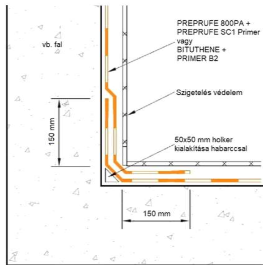
FÜGGŐLEGES BELSŐ SAROK
