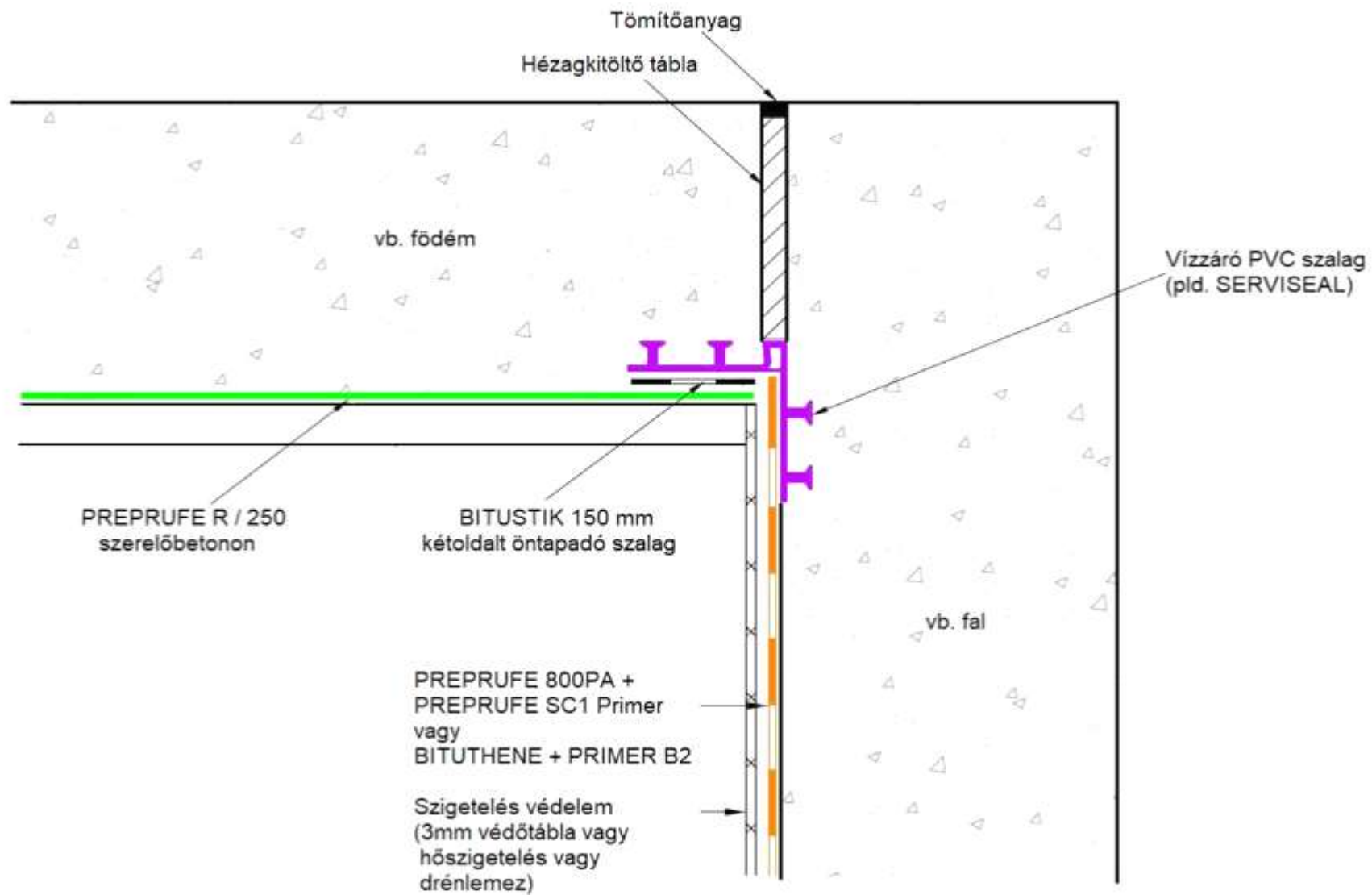
VB. FAL A VB. FÖDÉM FELSŐ SZINTJÉIG
