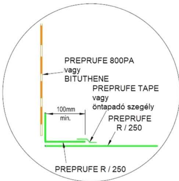
ALTERNATÍV PREPRUFE R / 250 KONFIGURÁCIÓ VÍZSZINTESBŐL FÜGGŐLEGESBE
