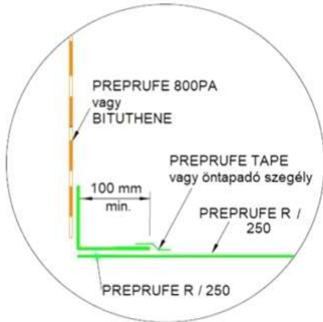
ALTERNATÍV PREPRUFE R / 250 KONFIGURÁCIÓ VÍZSZINTESBŐL FÜGGŐLEGESBE
