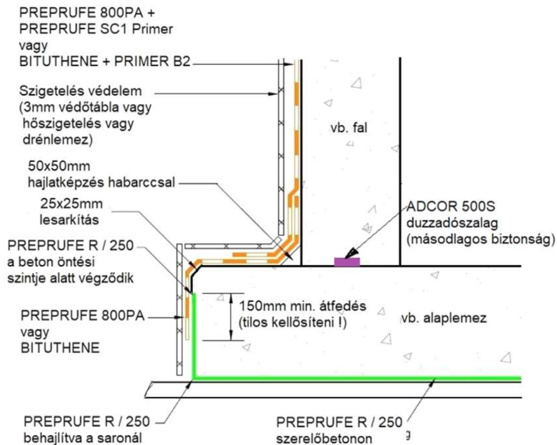
VASBETON FAL - KIUGRÓ VASBETON ALAPLEMEZ
