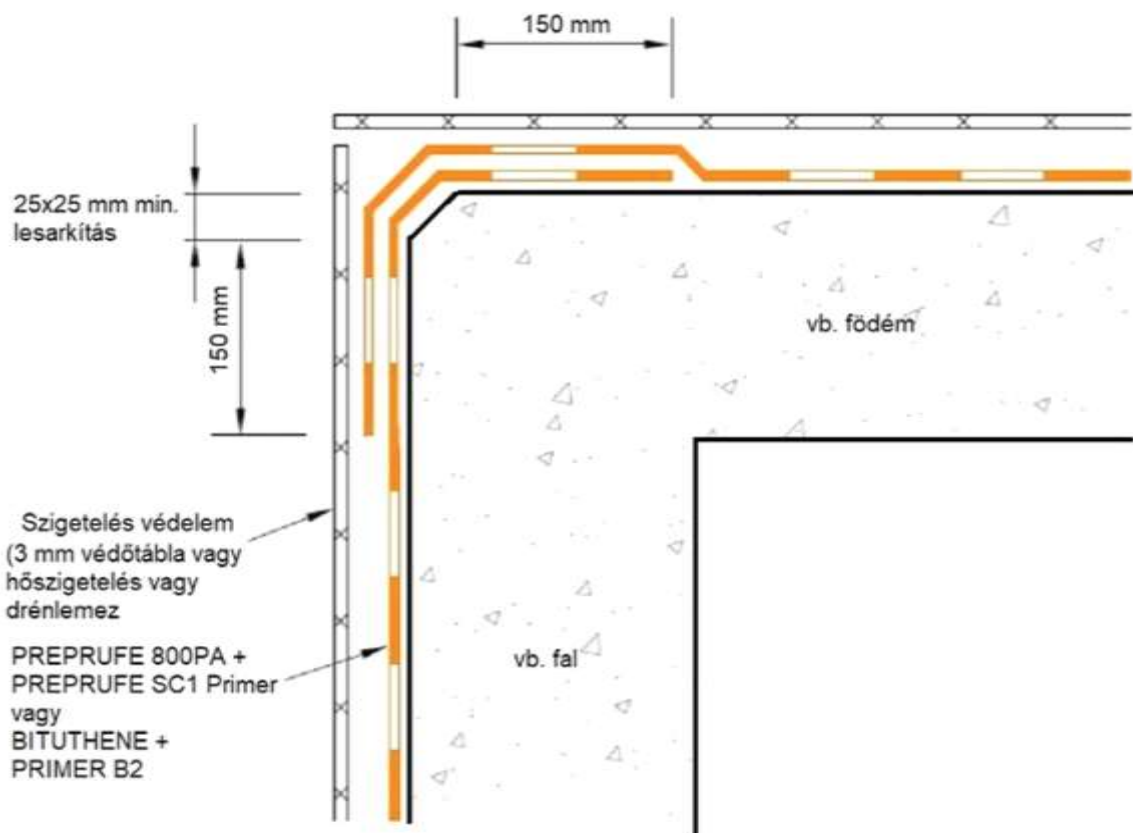
FÜGGŐLEGES KÜLSŐ SAROK
