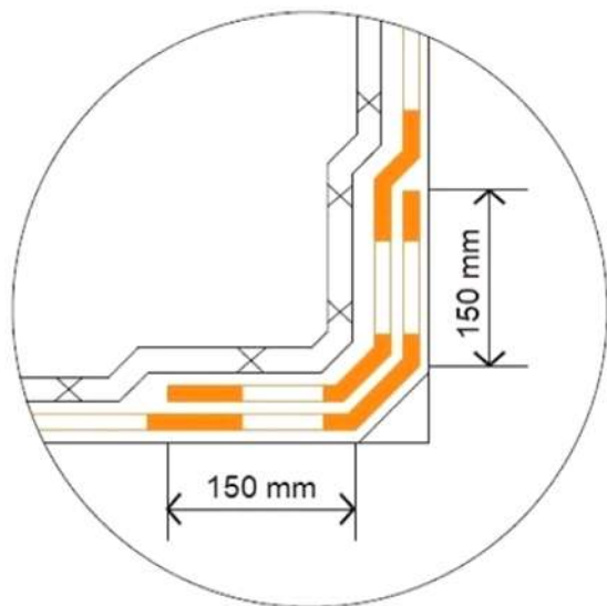
PREPRUFE 800PA / BITUTHENE KONFIGURÁCIÓ VÍZSZINTESBŐL FÜGGŐLEGESBE
